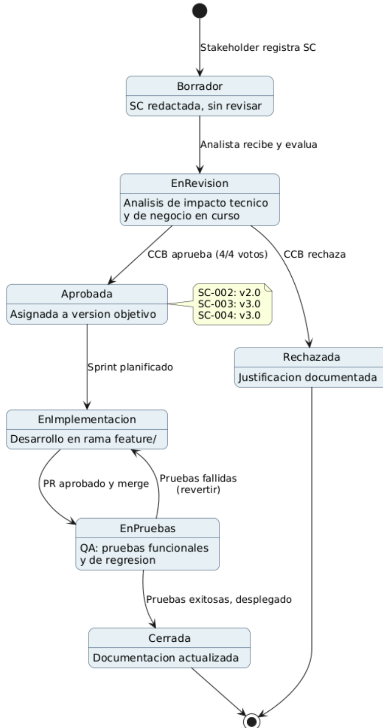
Figura 4.3.1b: Diagrama de Estado — Ciclo de Vida de una Solicitud de Cambio (SC)
