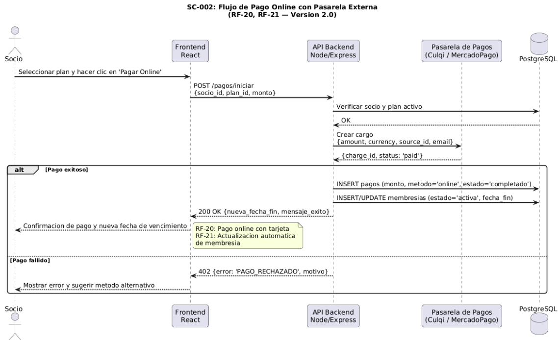
Figura 4.3.3: Diagrama de Secuencia — Integración con Pasarela de Pagos Online (SC-002)
