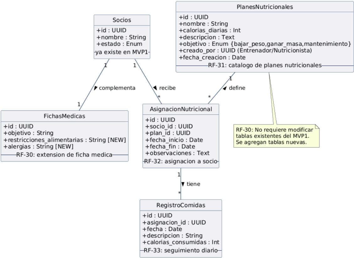
Figura 4.3.5: Diagrama de Clases — Modelo de Datos del Módulo Nutricional (SC-004, v3.0)
