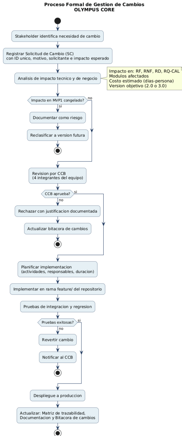
Figura 4.3.1: Diagrama de Actividad — Proceso Formal de Gestión de Cambios CCB
