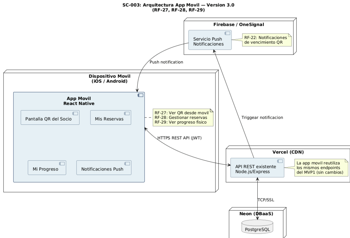
Figura 4.3.4: Diagrama de Componentes — Arquitectura App Móvil (SC-003, v3.0)
